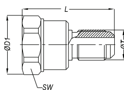
Male Thread Coupler (JIC 37°-SEA J514) Kupplung mit Aussengewinde (JIC 37°-SEA J514)
